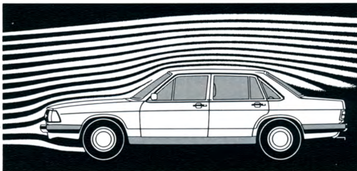
Die schöne stromungsgünstige Form des Audi 100 wurde im Windkanal ermittelt.
