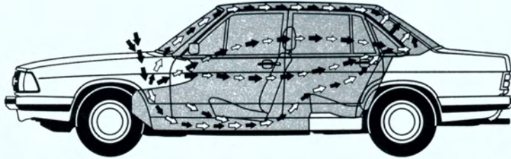
Das temperaturkonstante Heizungs- und Belüftungssystem mit Breitband-Luftströmung und Schnellregel-Effekt. Oben angenehm kühl. Unten behaglich warm.
